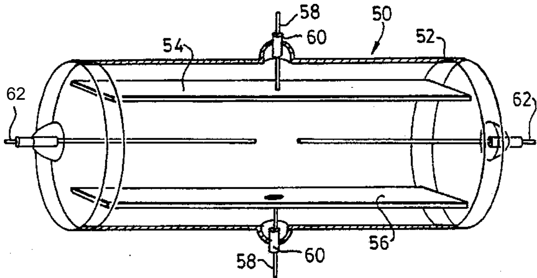
Abbildung 2-2: Aufbau der PAGD-Gasentladungs-Röhre nach Correa (Quelle: Patent 5,416,391)
